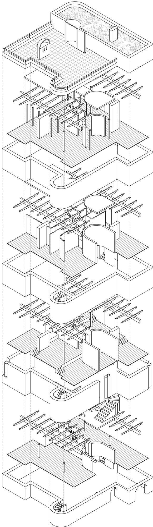
Axonometrie
